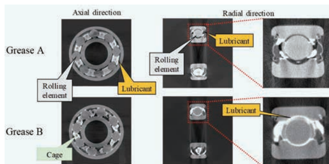
図 2. 軸受回転試験後の中性子 CT 観察 3
