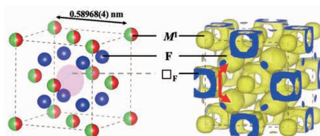
図 5. 573 K における \text{Ca}_{0.48}\text{Ba}_{0.52}\text{F}_2 固体電解質 ( M' = \text{Ca}_{0.48}\text{Ba}_{0.52} ) の結晶構造 (左) と核密度分布 (右)。赤線は「 \text{F}-\square_F-\text{F} 」間を結ぶフッ化物イオン伝導経路。 \square_F は格子間サイトに相当する。
