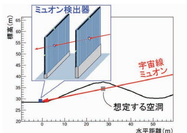
図4. 古墳を透過したミュオンの捕まえ方
