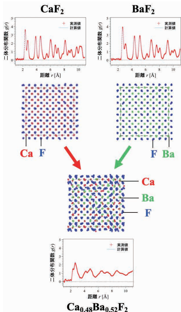
図6. \text{Ca}_{0.48}\text{Ba}_{0.52}\text{F}_2 固体電解質および \text{CaF}_2 、 \text{BaF}_2 のRMCモデリングの結果と原子配列(室温)。
