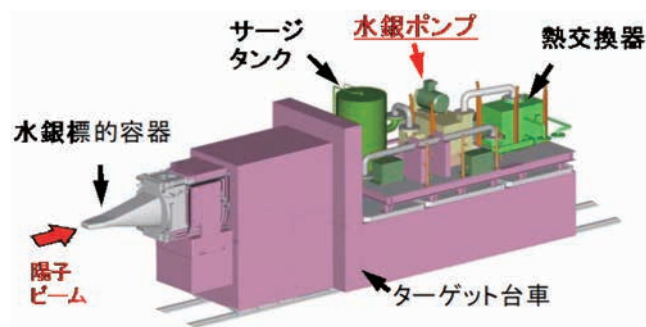
図1. 水銀循環系概要
