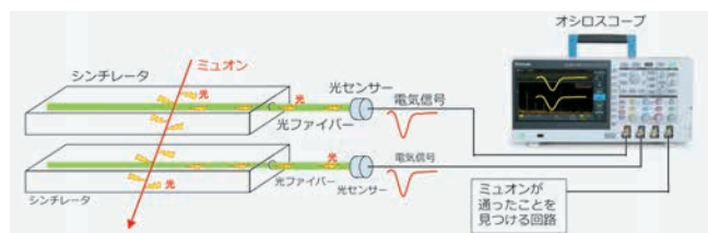
図7. 測定原理
