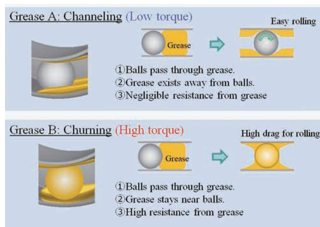
図 4. 各グリースの潤滑機構のイメージ 3
