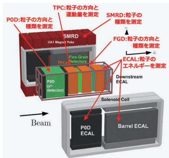
図6a. T2K前置検出器(置き換え前)とPOD測定器の役割
