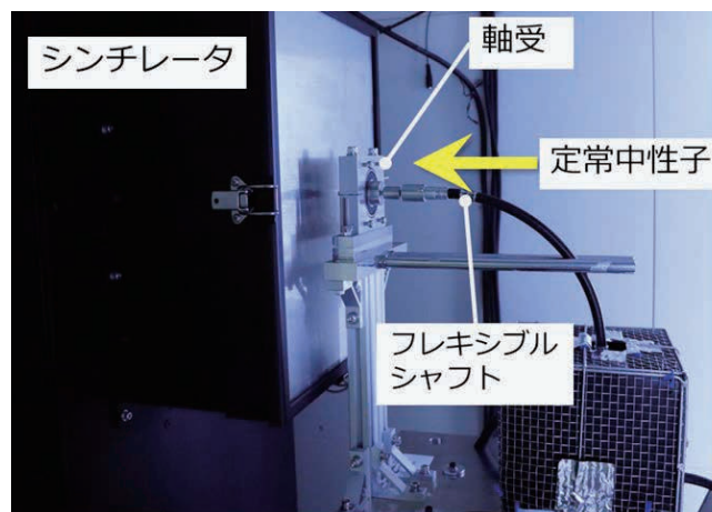
図 1. 軸受回転中の中性子イメージング観察方法
