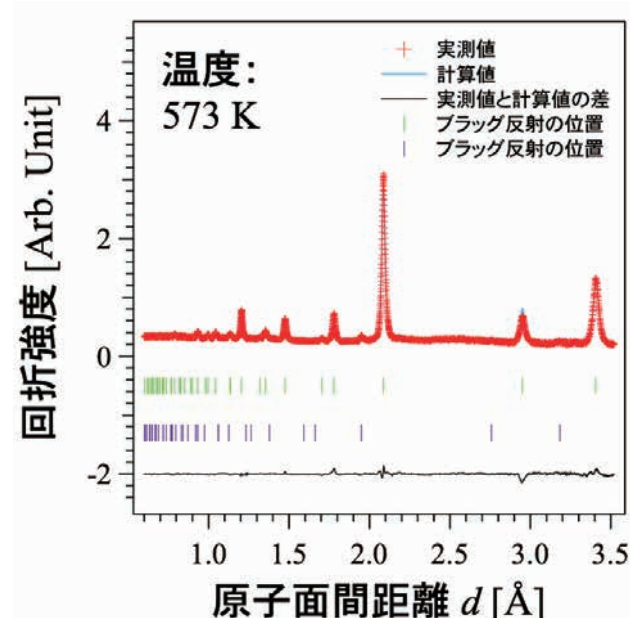
図 4. \text{Ca}_{0.48}\text{Ba}_{0.52}\text{F}_2 固体電解質のリートベルト解析の結果 (573 K)。緑の縦棒は \text{Ca}_{0.48}\text{Ba}_{0.52}\text{F}_2 相 (主相)、紫の縦棒は微量の副相 (2% 以下) を表している。
