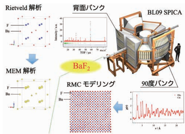
図 1. BL09 SPICA の概要。背面バンクおよび 90 度バンクで測定した \text{BaF}_2 の回折データ。背面バンクではリートベルト法および最大エントロピー法 (MEM) による解析例、90 度バンクでは二体分布関数 (PDF) データを用いた逆モンテカルロ (RMC) モデリングによる解析例を示している。
