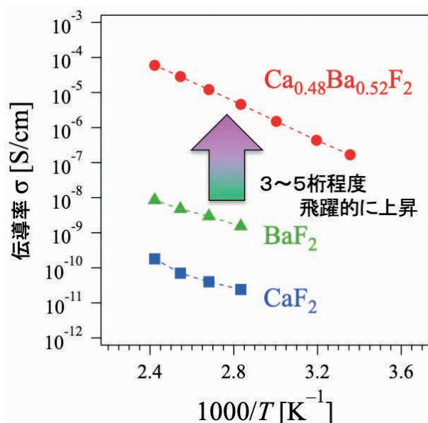
図 3. \text{Ca}_{0.48}\text{Ba}_{0.52}\text{F}_2 固体電解質および \text{CaF}_2 、 \text{BaF}_2 のイオン伝導率の温度変化。
