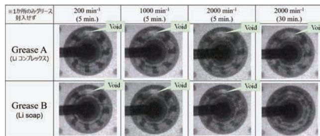
図 3. 軸受回転中の中性子ラジオグラフィー観察
