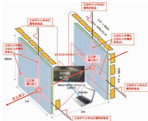
図9. 飛跡検出の原理
