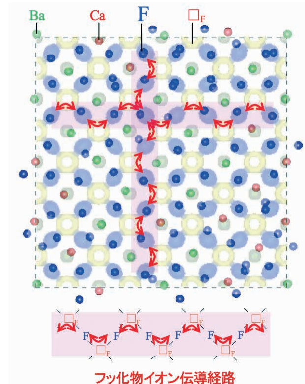
図7. \text{Ca}_{0.48}\text{Ba}_{0.52}\text{F}_2 固体電解質のフッ化物イオン伝導経路と原子配列の乱れを重ね合わせたイオンの流れのイメージ図。赤線は「 \text{F}-\square_{\text{F}}-\text{F} 」間を結ぶフッ化物イオン伝導経路。
