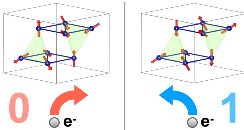
図3：反強磁性体 \text{CoTa}_3\text{S}_6 、 \text{CoNb}_3\text{S}_6 において実現している四面体状の非共面なスピン配列。2種類のスピン状態は、それぞれ逆符号のトポロジカルホール効果を生じるため、電気的に区別して読み出すことが可能となる。
