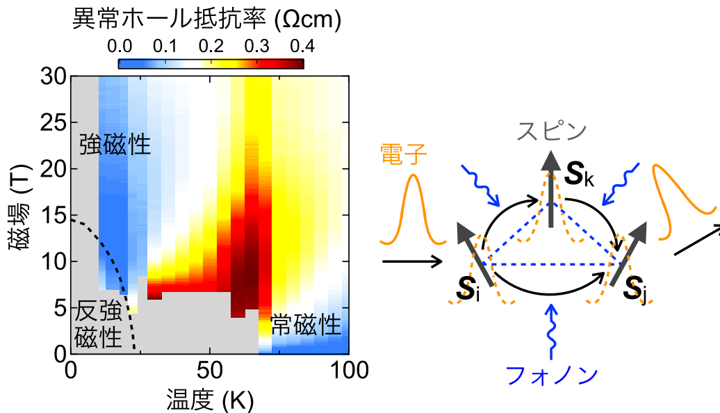
図 3. (左)磁化に比例しない異常ホール抵抗成分の温度磁場相図上の強度。(右)有限のスピンのカイラリティを持つ非共面的なスピンの配置におけるホッピング伝導を考慮した異常ホール効果の理論。
